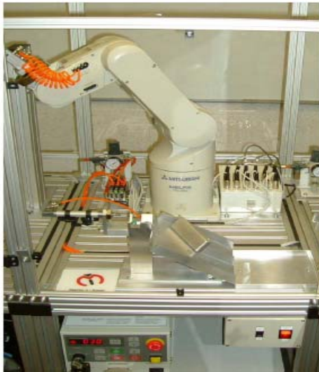
Roboter Prüfstation
