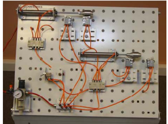
Pneumatischer Schaltplan
